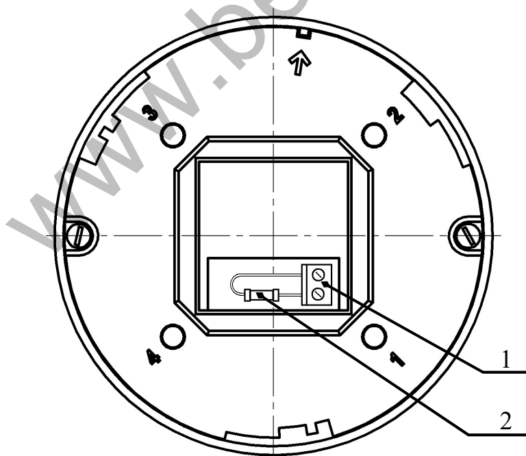
Рис. 2 Установка ограничивающего резистора R_{огр} .
