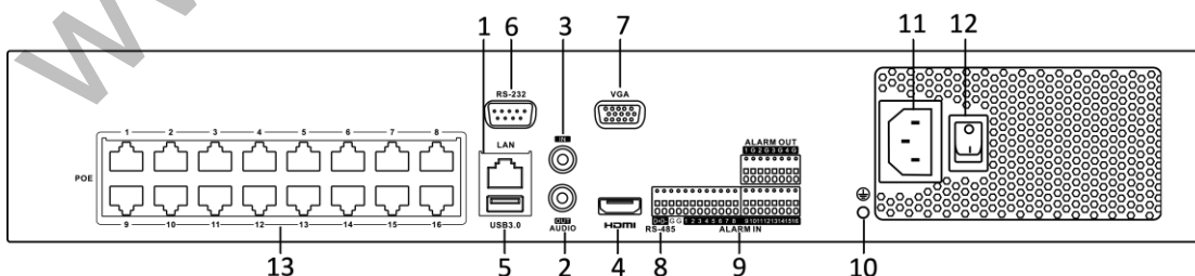
Рисунок 1-17 Серии DS-7700NI-I4/16P и DS-7700NI-K4/16P
