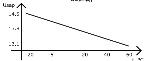
Графік температурної стабілізації напруги заряду
