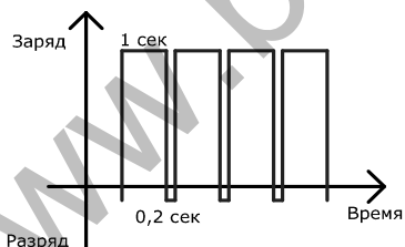
Час заряду АКБ (12V)
