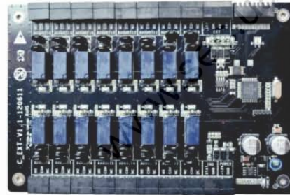
EX16 Плата расширения
