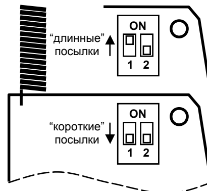
Рис.2. Переключение радиокнопки в режим «длинные посылки»
