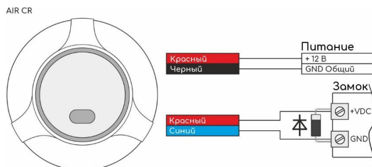
Рисунок 8. Использование защитного диода
