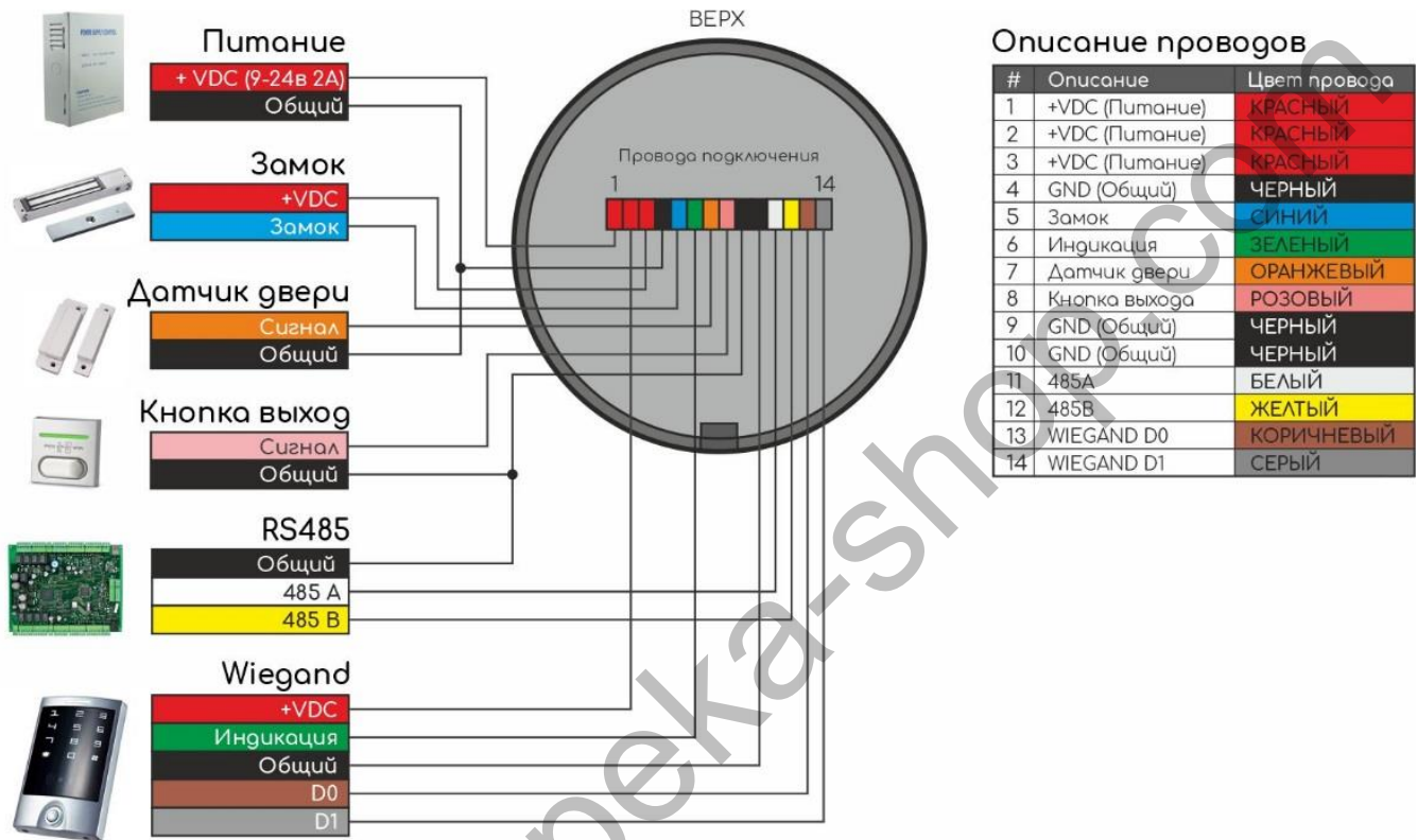
Рисунок 1 – Цветовое обозначение проводов интерфейса
