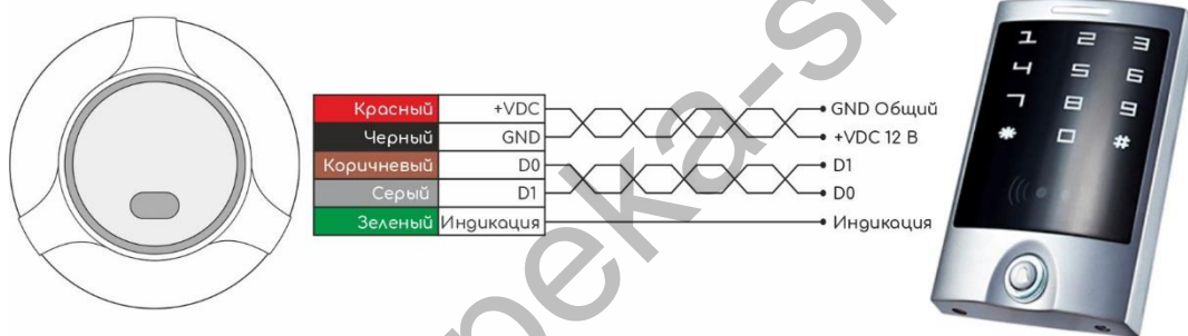
Рисунок 7. Рекомендуемая схема подключение по интерфейсу Wiegand
