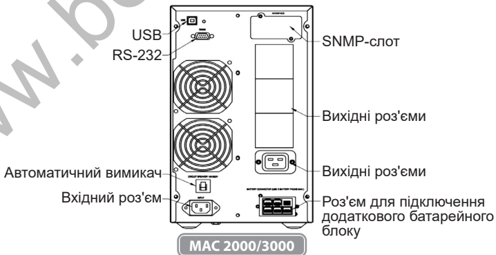
Мал.4. Задня панель серії MAC
