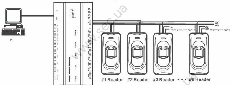
Соединение между InBio460 и считателями InBio
