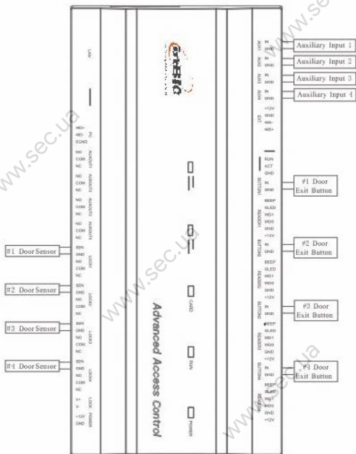
Пример соединения между InVio460 и внешними аксессуарами
