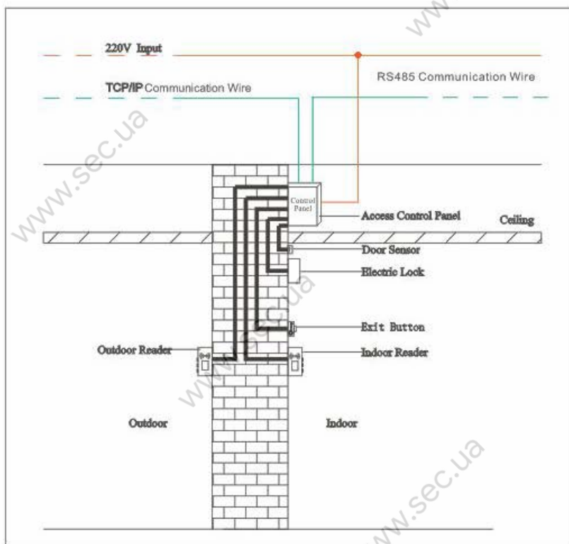
Подключение проводов
