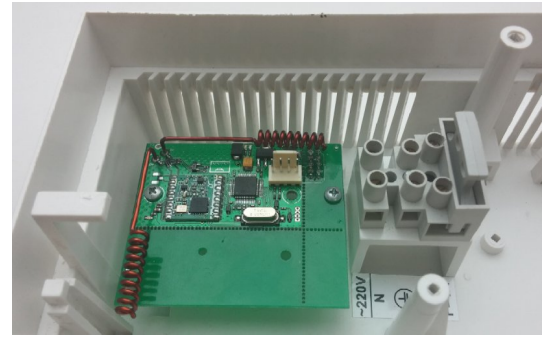
Рисунок 31. Радиоприемник Ajax «uartBridge» в корпусе прибора
