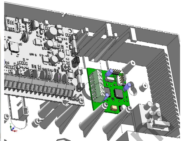
Рисунок 35. Установка модуля «Дозор»
