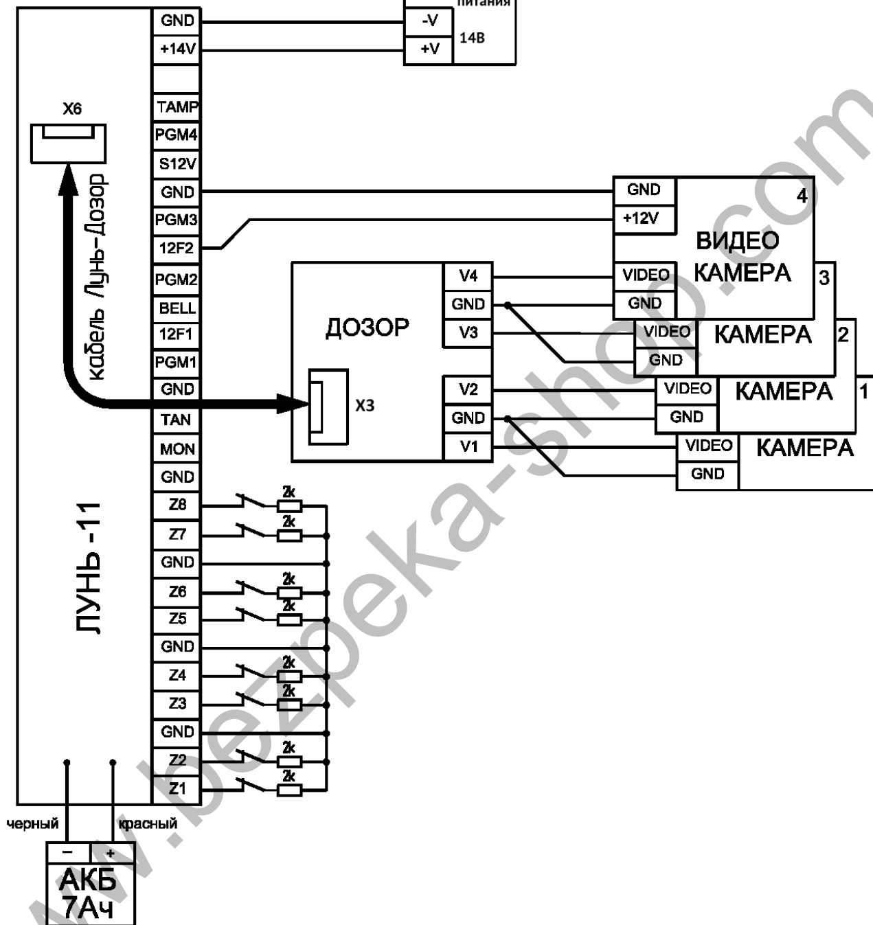
Рисунок 44. Схема подключения модуля фотоподтверждения тревог «Дозор»
