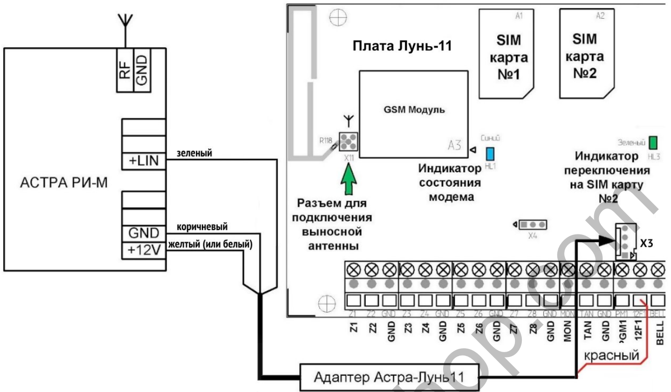
Рисунок 45. Схема подключения РПУ «Астра RI-M»
