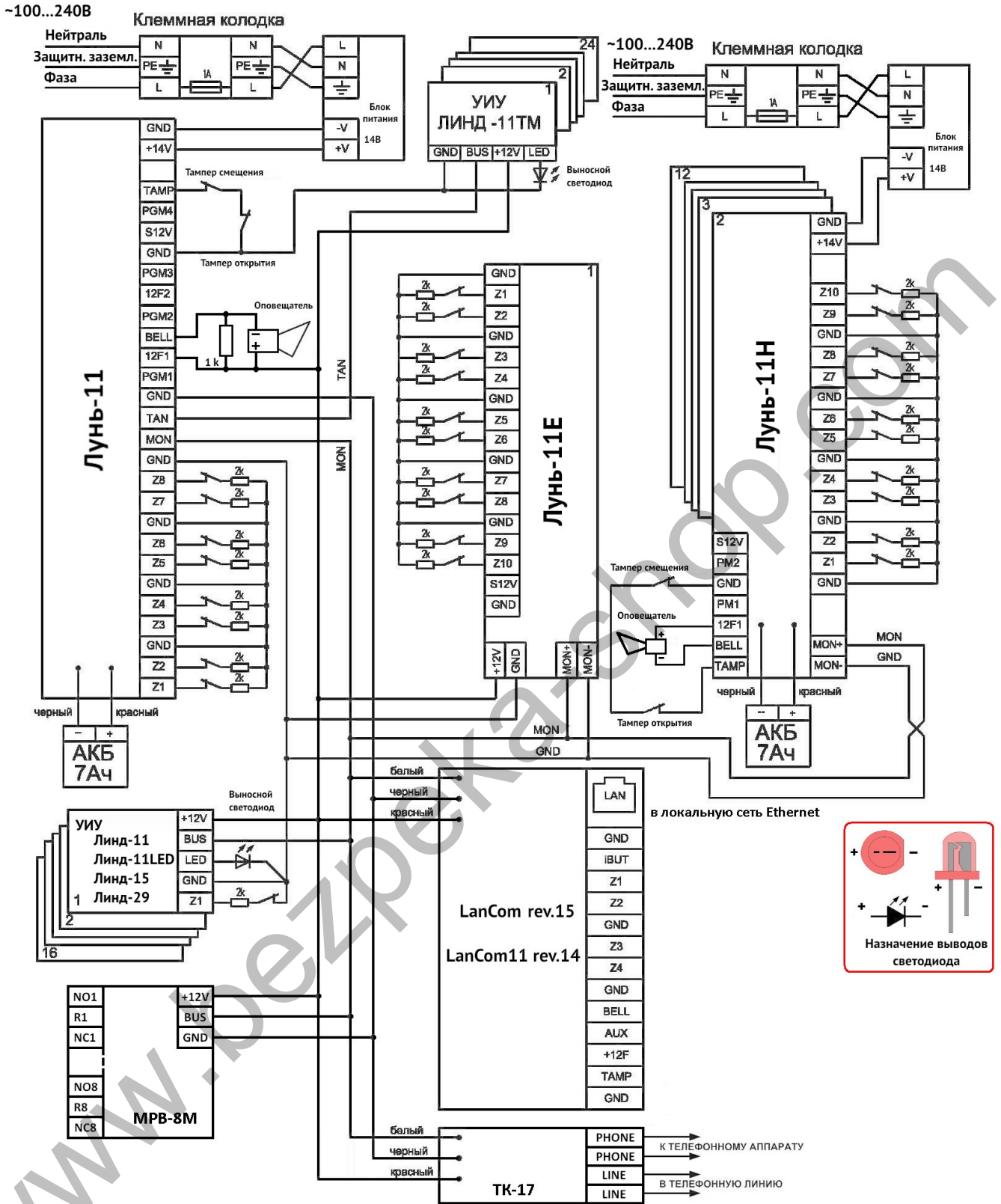
Рисунок 43. Схема подключения сетевых устройств
