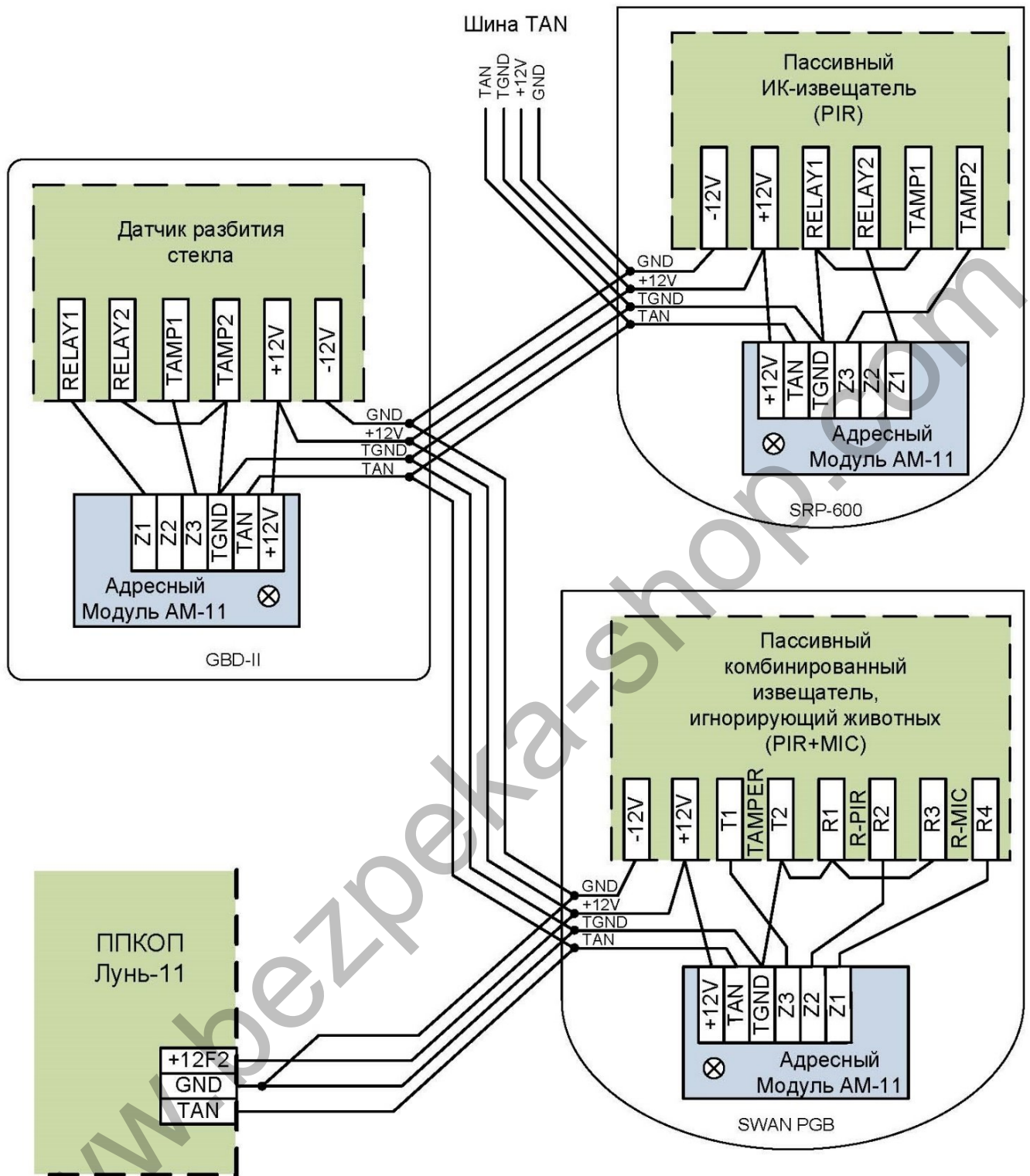
Рисунок 42. Пример использования адресных модулей «АМ-11»
