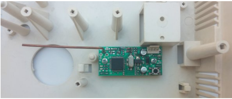
Рисунок 30. Радиоприемник Ajax «RR-108» в корпусе прибора
