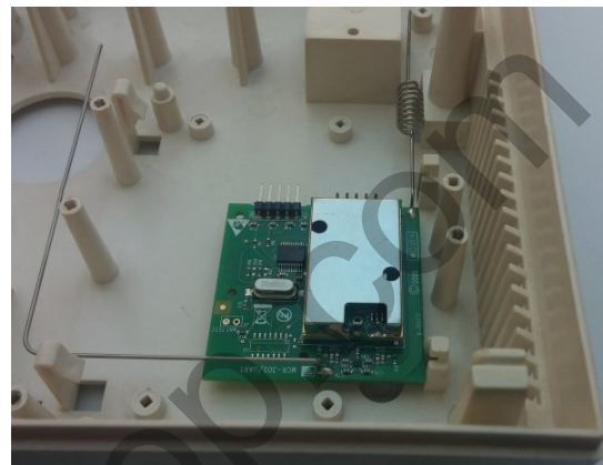
Рисунок 23. Радиоприемник «MCR-300» Visonic в корпусе прибора
