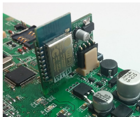
Рисунок 38. Установка модуля «W11M» в X6
