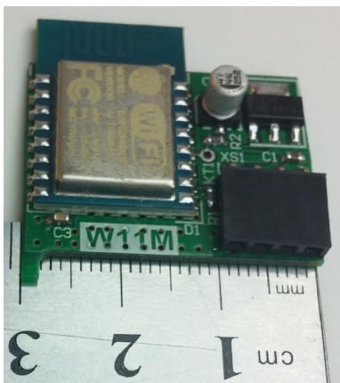
Рисунок 36. Общий вид модуля «W11M»
