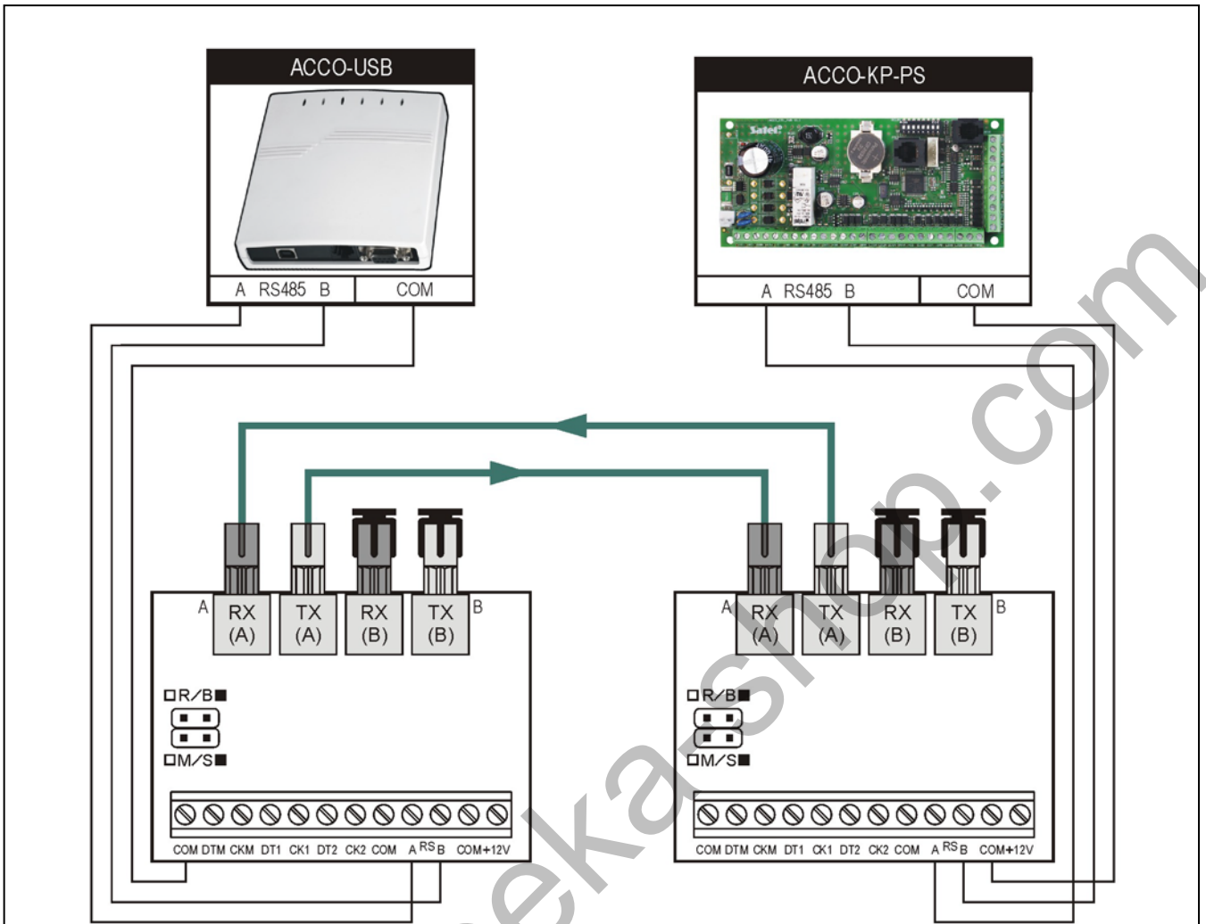
Рис. 4. Пример работы двух конвертеров INT-FI, подключенных к магистрали RS-485 СКУД ACCO. В конвертерах перемычки сняты. Питание конвертера, подключенного к контроллеру ACCO-KP-PS, может осуществляться от платы модуля. Питание и второго конвертера может осуществляться от независимого источника питания (БП) локально.
