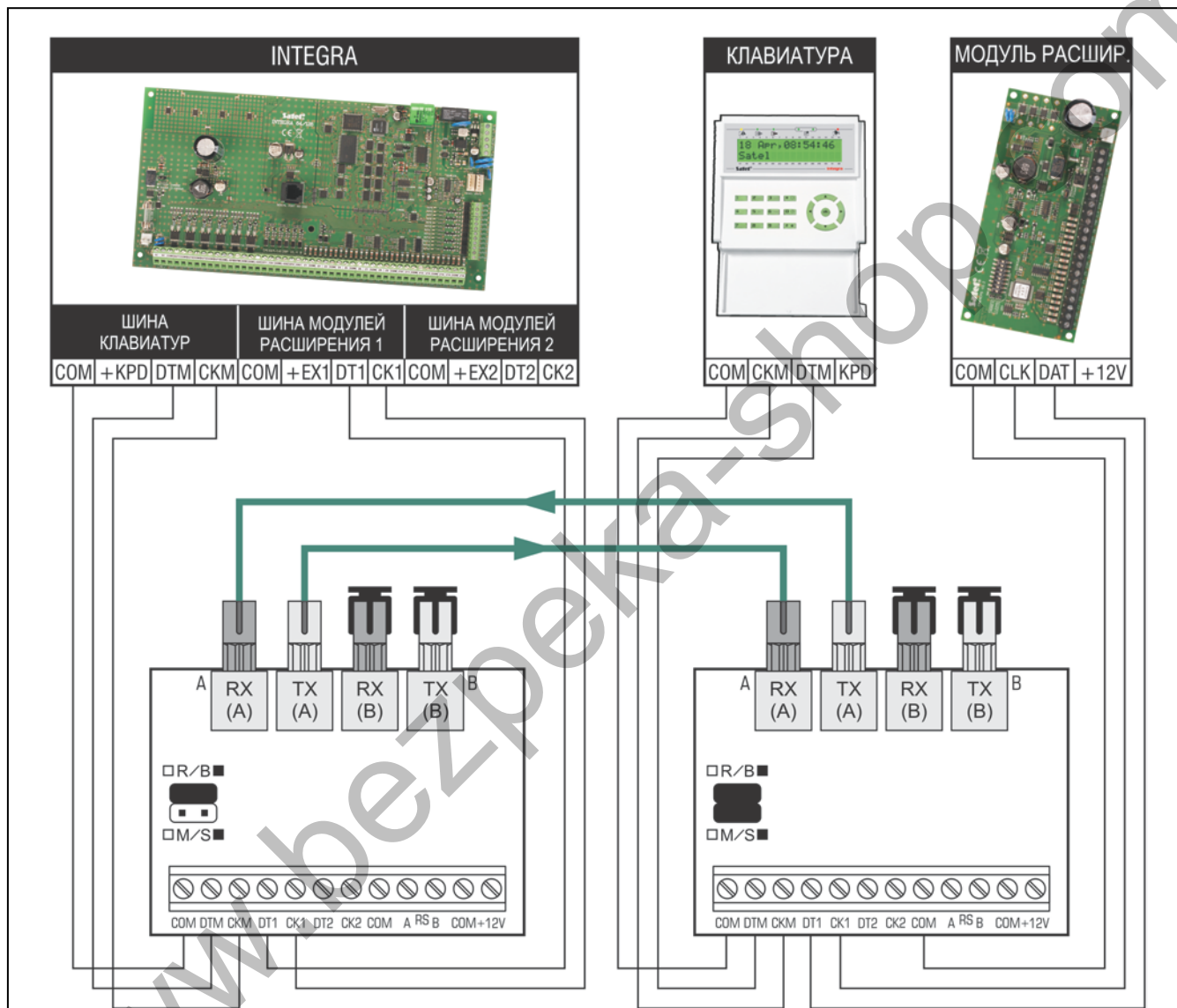
Рис. 3. Пример работы двух конвертеров INT-FI, подключенных к ПКП INTEGRA. Конвертер, подключенный к ПКП в конфигурации Master (переключки M/S снята), конвертер, подключенный к клавиатуре или модулю расширения – в конфигурации Slave (переключки M/S установлена). Питание конвертера, подключенного к ПКП, может осуществляться от главной платы ПКП. Питание второго конвертера может осуществляться от независимого источника питания (БП, модуль расширения с БП). К конвертеру, работающему в конфигурации Slave, можно подключить большее число клавиатур и модулей расширения, чем указано на рисунке.
