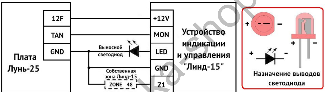
Рисунок 23. Схема подключения УИУ к ППКОП «Лунь-25»
