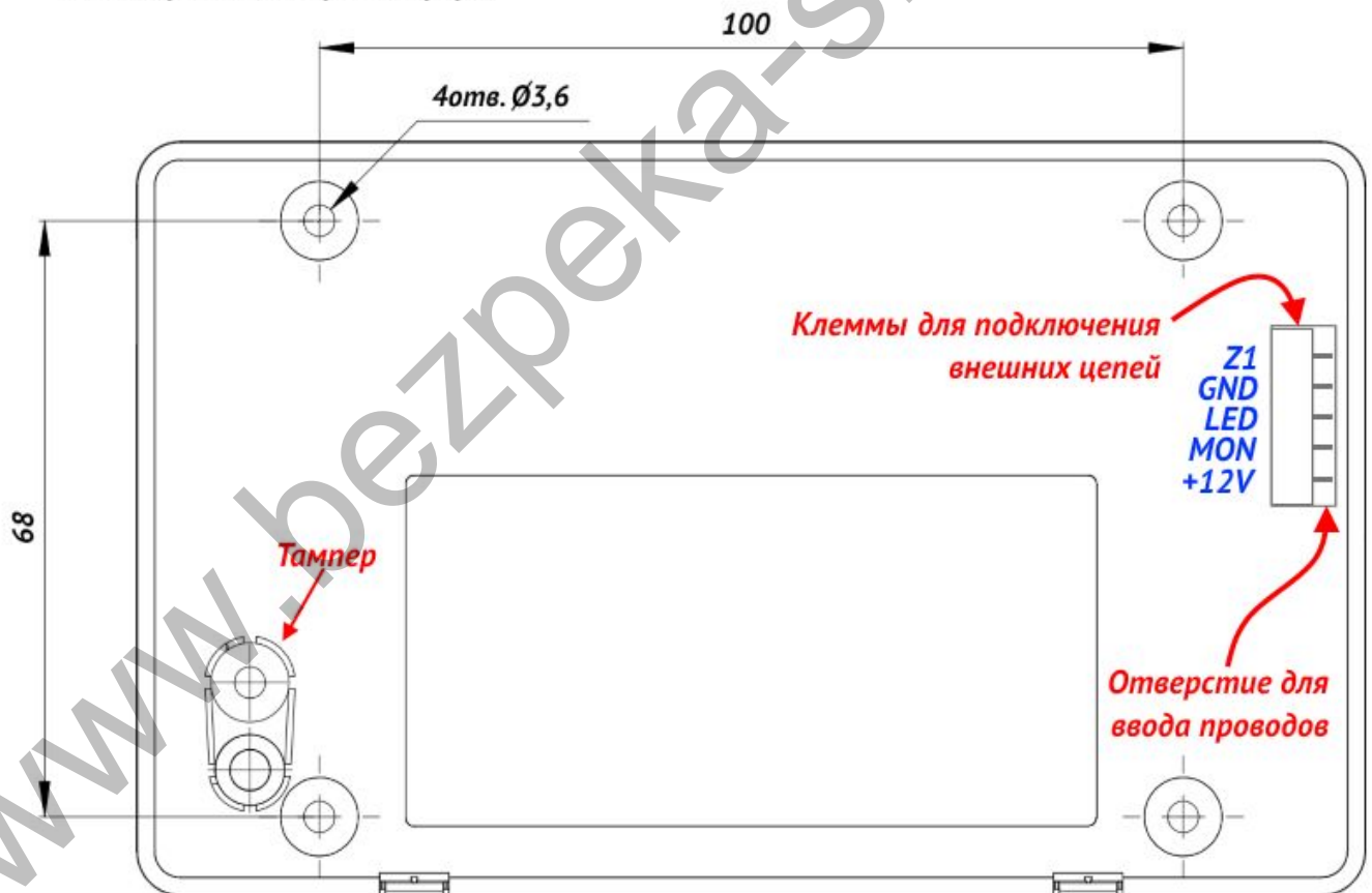
Рисунок 3. Внешний вид с обратной стороны корпуса и установочные размеры
