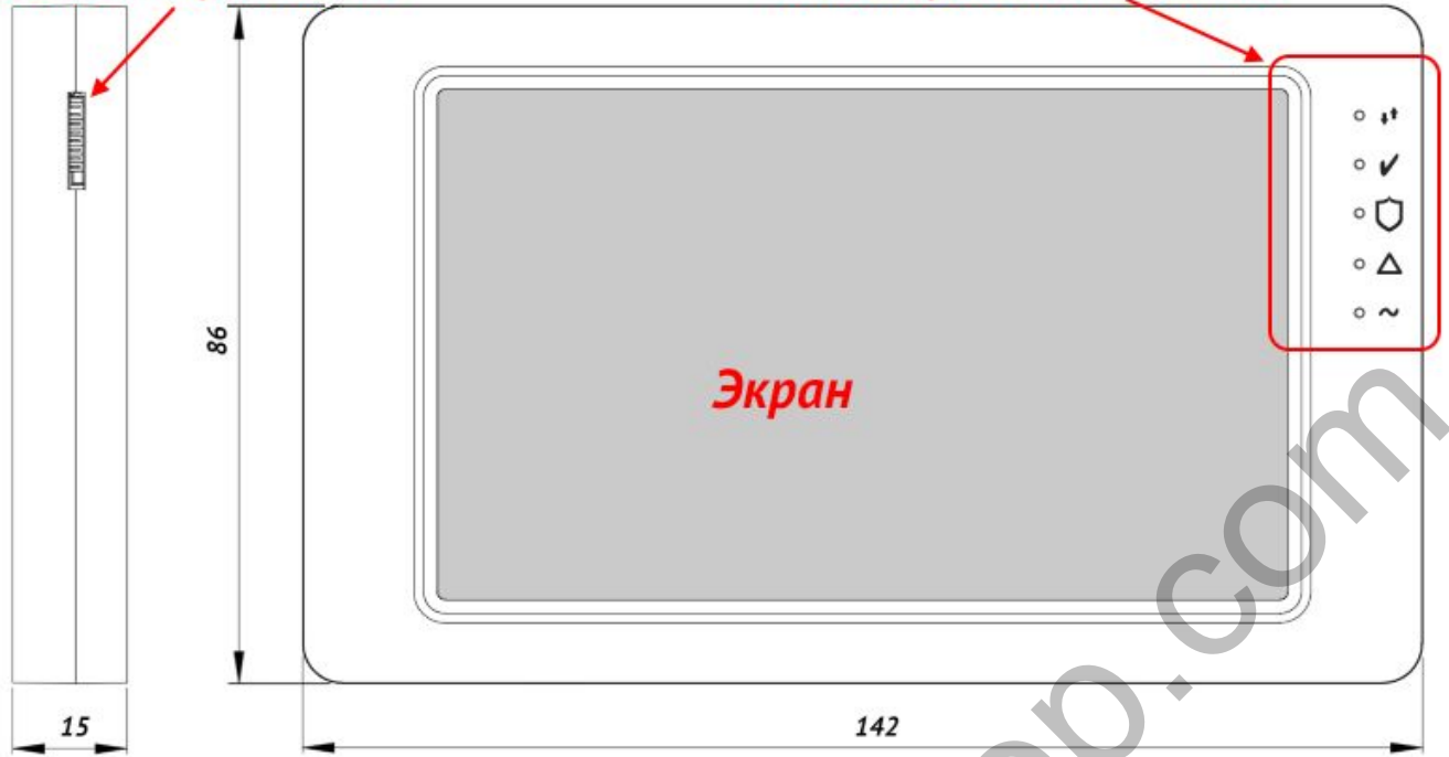
Рисунок 2. Габаритные размеры УИУ "Линд-15"
