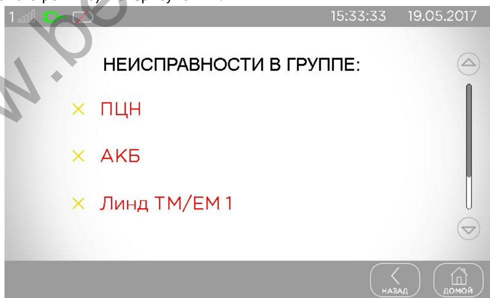
Рисунок 11. Экран неисправностей
