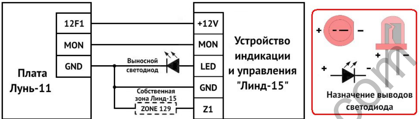
Рисунок 22. Схема подключения УИУ к ППКОП «Лунь-11»
