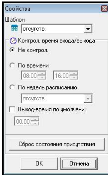
Рис. 37. Окно СВОЙСТВА.
