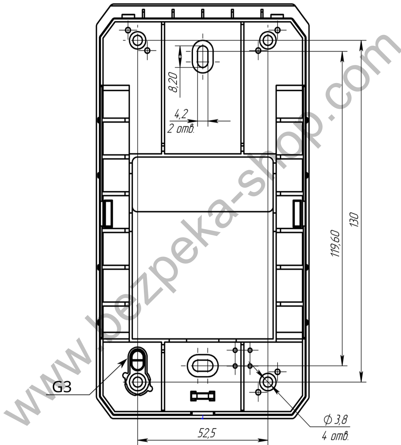
Рисунок 1 – Установчі розміри клавіатури
